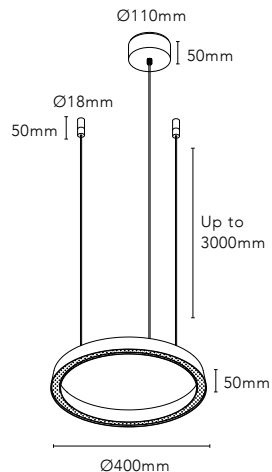
EDGE ROUND Ø400
